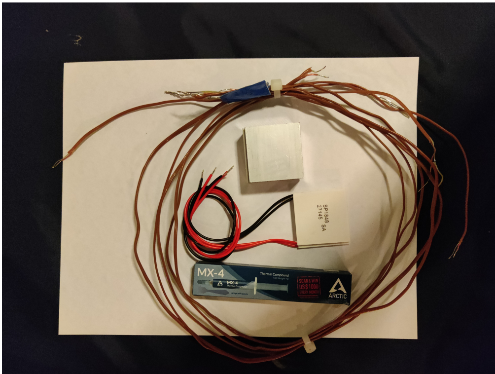
Fig6. TEG Subsystem
